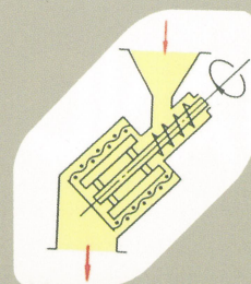
RDG型サニタリードレッサー GMP適合の無菌チェックふるい
