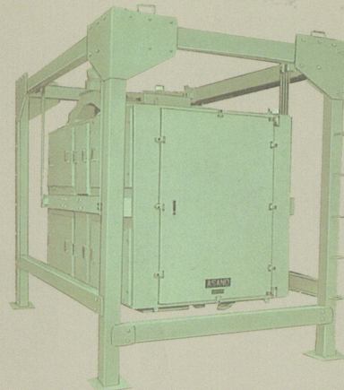
STHD-35型プランシフター 70型と同構造で、ふるい網面積が2分の1
